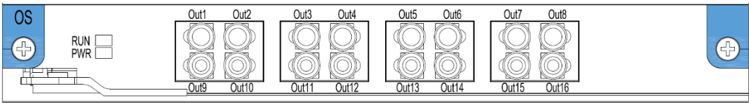
图 2-5 光源板卡效果图
