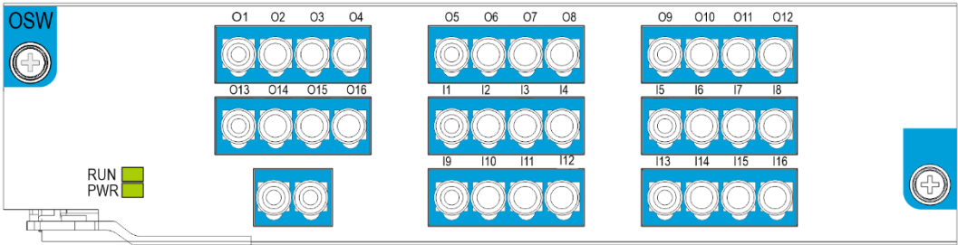
图 2-10 矩阵光开关效果图
