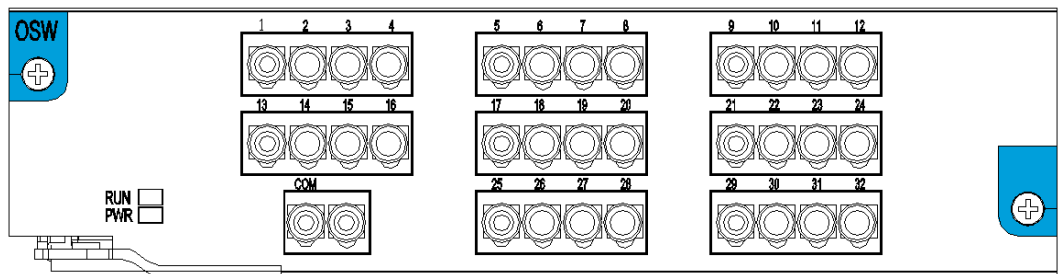
图 2-3 光开关板卡效果图
