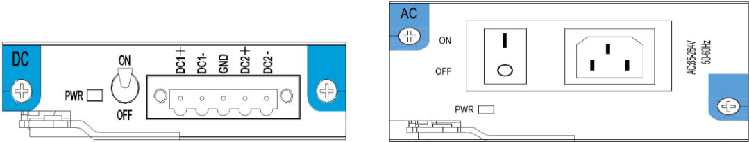
图 2-2 电源板卡效果图
